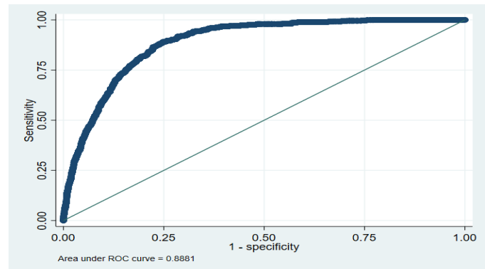
Graphique 2 courbe ROC
